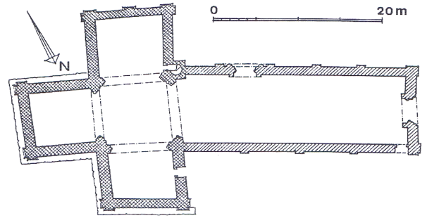
Plan de l'église partiellement fortifiée (G. Redelius)
